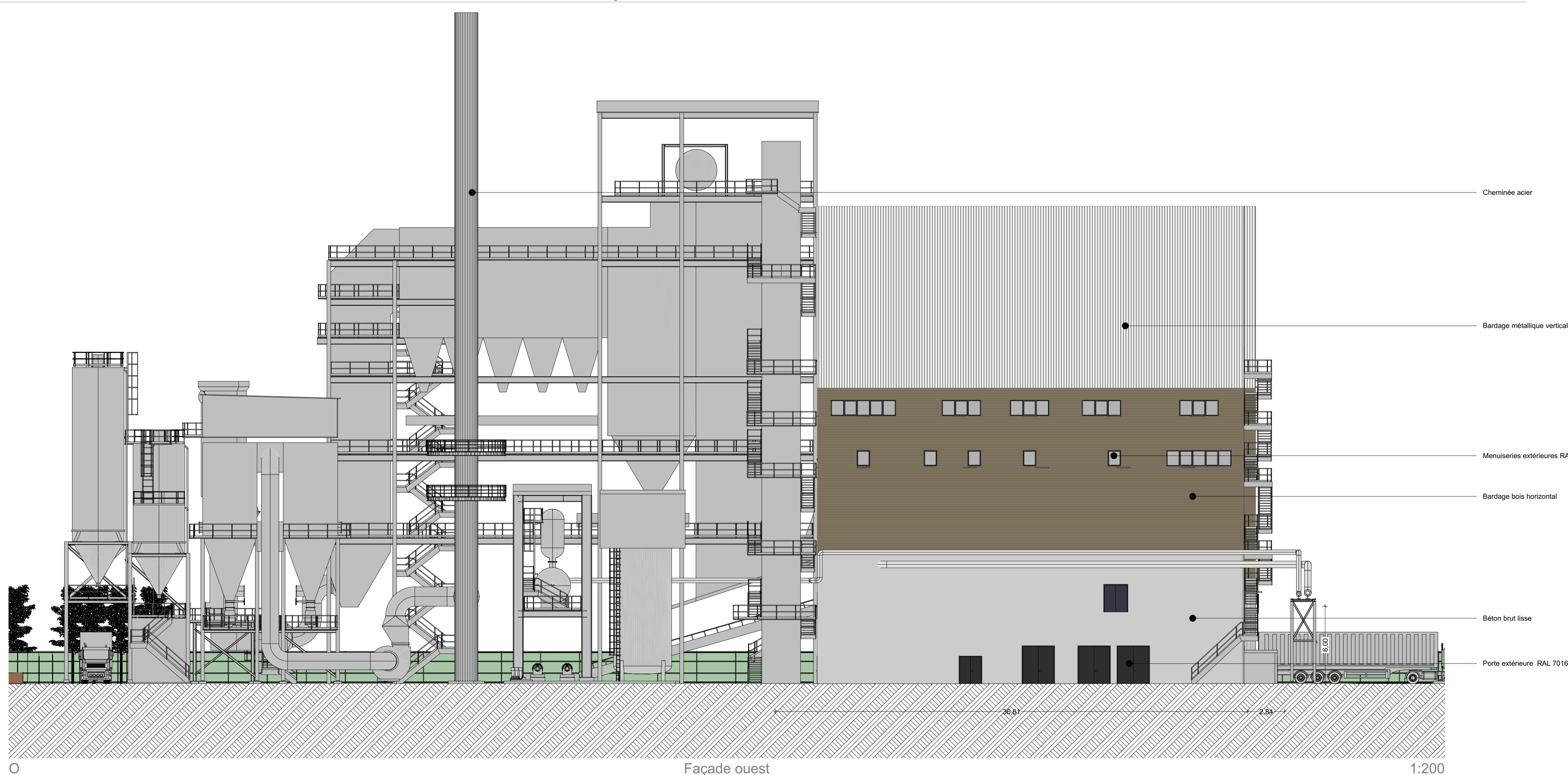
Façade ouest
