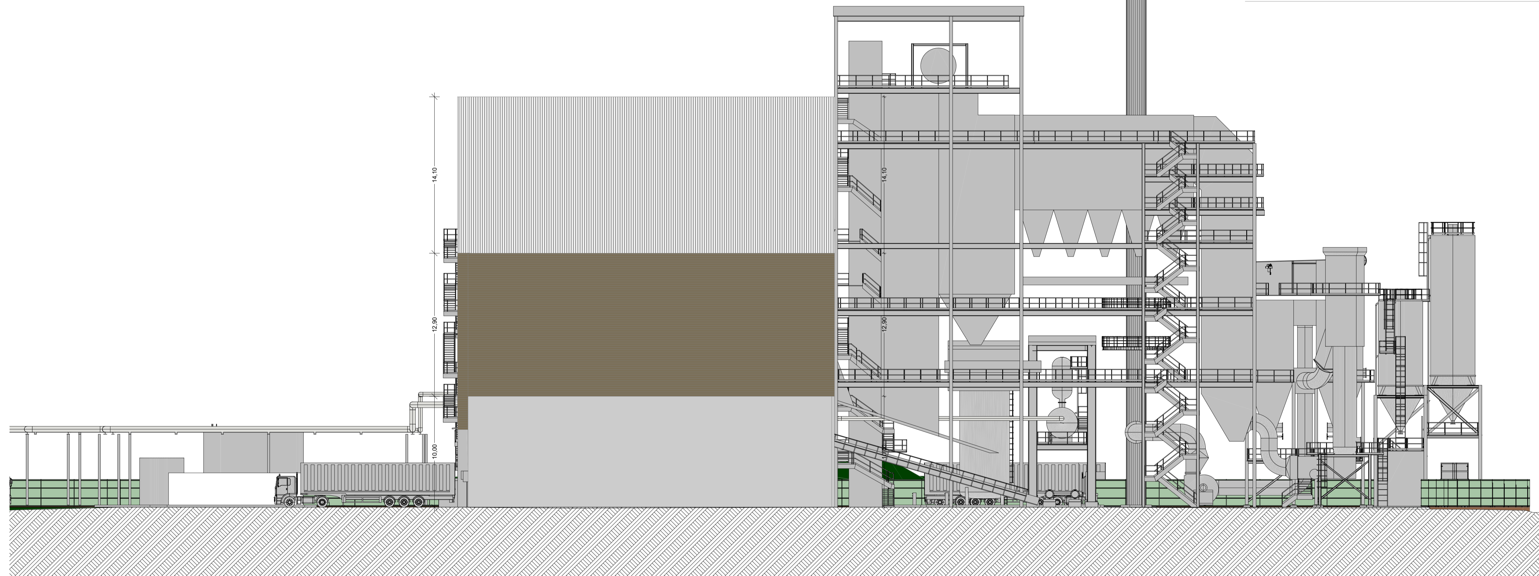
Façade est
