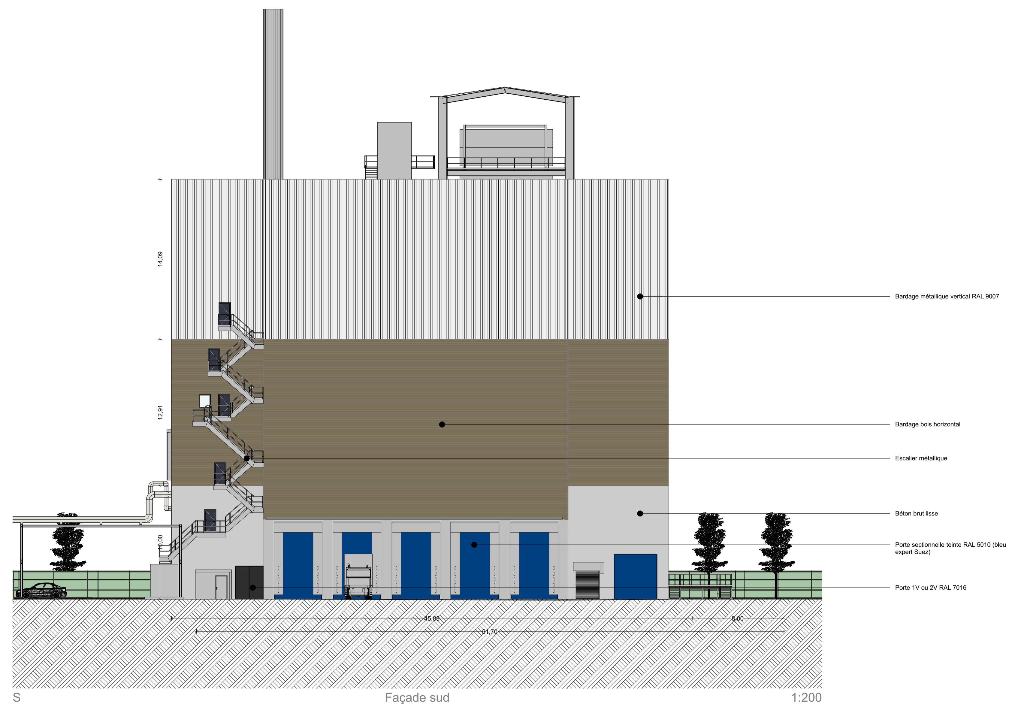
Façade sud
